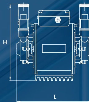
TWIN IMPELLER PUMPS - STP-1.5 B, STP-2.0 B, STP-3.0 B, STP-4.0 B
